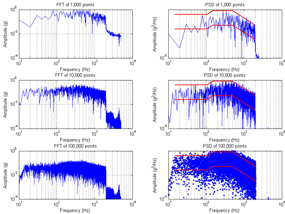
شکل ۱ نمونه تحلیل انجام شده بر روی دیتای خام
