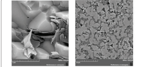
تصاویر میکروسکوپ الکترونی روی از سطح پولیش شده و مقطع شکست کامپوزیت بوریدی-کاربیدی-نیتريدی
